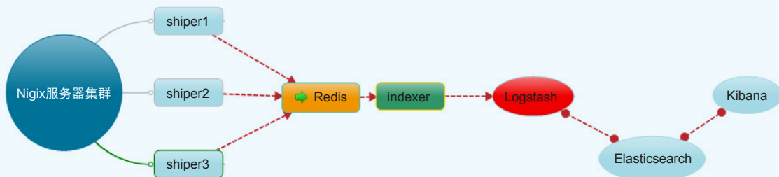
图1 国家气象业务内网ELK实时日志分析系统的架构图
